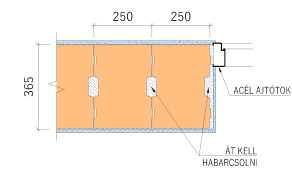
- KÖTÉS AZ AJTÓFALAZATNÁL, AZ 1. SOR FALAZAT
