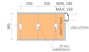
- KÖTÉS AZ AJTÓFALAZATNÁL, A 2. SOR FALAZAT
