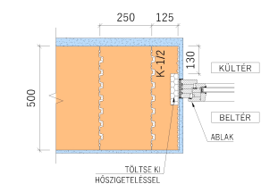
- KÖTÉS AZ ABLAKFALAZATNÁL, A 2. SOR FALAZAT
