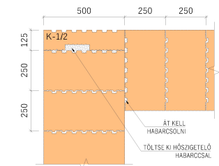
- SAROKKÖTÉS, A 2. SOR FALAZAT
