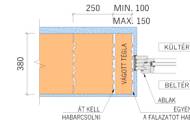
- KÖTÉS AZ ABLAKFALAZATNÁL, A 2. SOR FALAZAT
