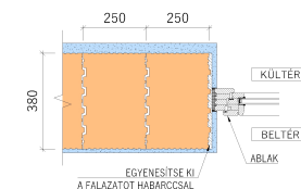
- KÖTÉS AZ ABLAKFALAZATNÁL, AZ 1. SOR FALAZAT
