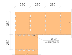
- SAROKKÖTÉS, A 2. SOR FALAZAT
