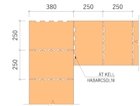
- SAROKKÖTÉS, AZ 1. SOR FALAZAT
