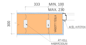
- KÖTÉS AZ AJTÓFALAZATNÁL, A 2. SOR FALAZAT
