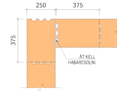
- SAROKKÖTÉS, AZ 1. SOR FALAZAT
